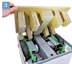
①自律移動ロボット【KeiganALI(ケイガンアリ)】。 ②従来の梱包はアルミケース+ウレタンを使用されていました。 ③初期のご提案では、積層ダンボールを用いての緩衝設計を検討いたしました。 ④商品の重量と紙の強度、コスト面を考え、最終では底面にウレタン+ダンボールで梱包することになりました。
